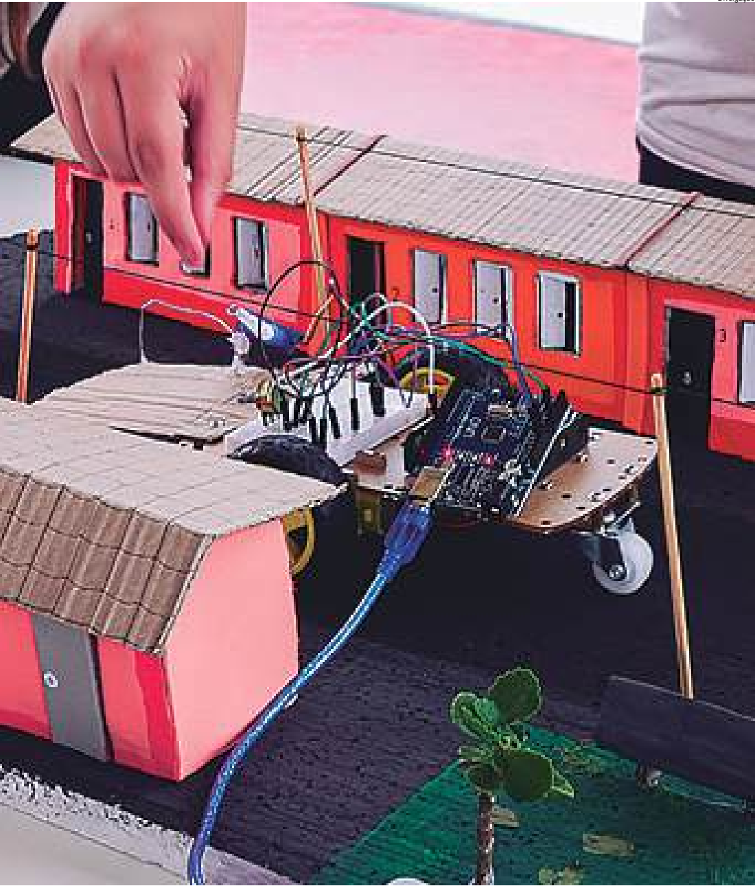
Protótipo Carrinho com Rampa de Acessibilidade
