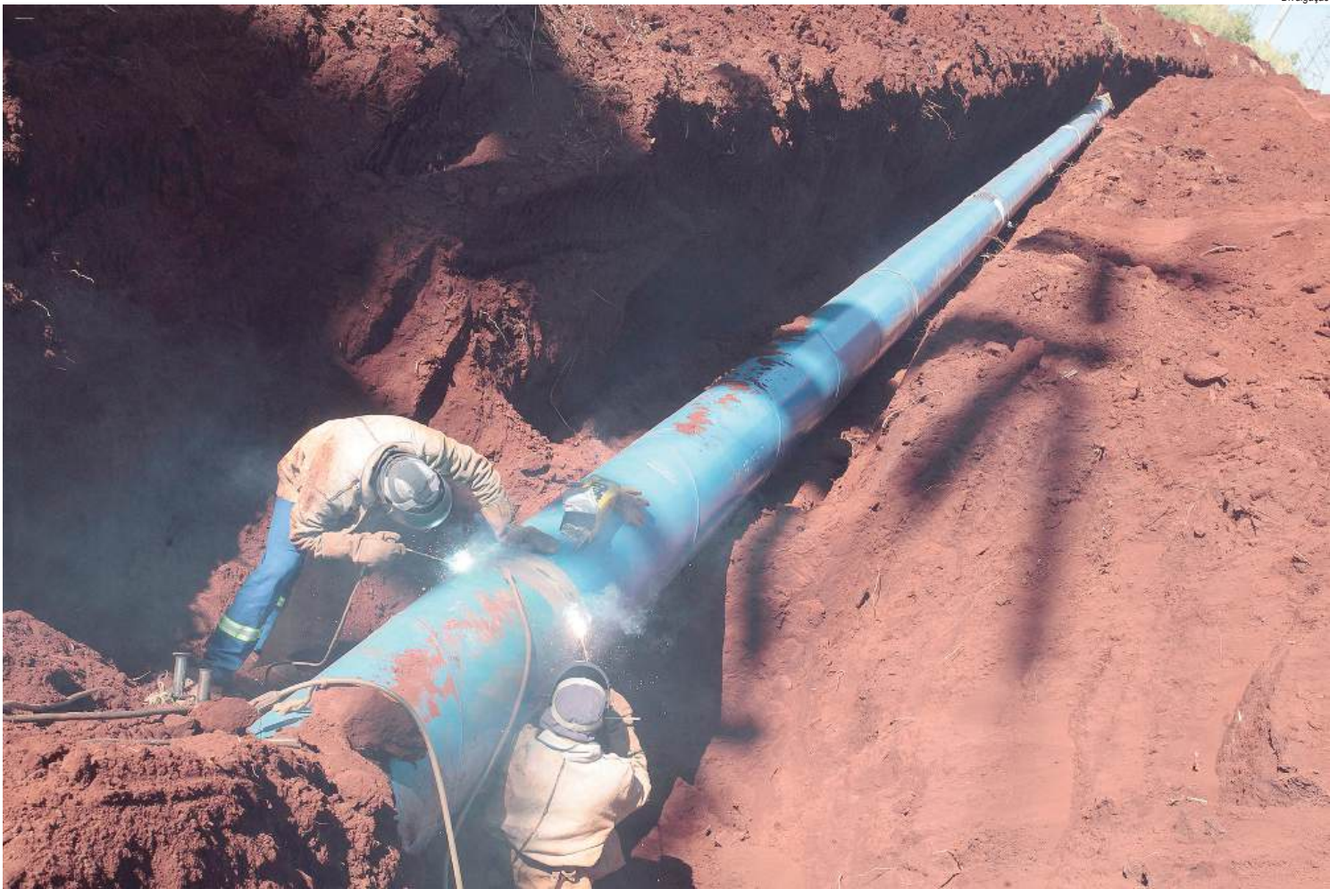
Equipes fazem a soldagem da tubulação da nova rede Torre de TV - Unileste
